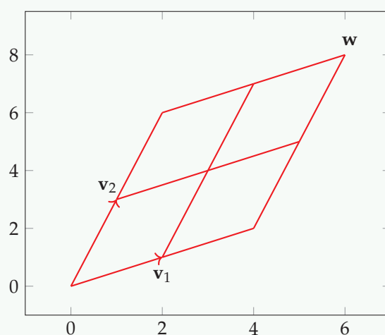
Figur 9.5: \beta -koordinaterne for \mathbf{w} er \begin{bmatrix} 2 \\ 2 \end{bmatrix} .
