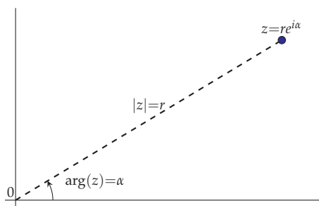
Figur 4.7: Det komplekst tal z skrevet på polær form.
